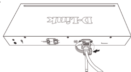
Figure 3-4. Faites tourner le collier du cordon d'alimentation
