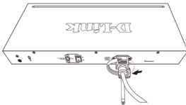
Abbildung 3-4. Stromkabel umwickeln
