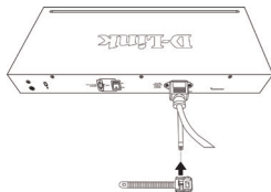
Figura 3-3. Deslize o retentor através da braçadeira
