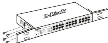
圖 2. 固定機架固定架
