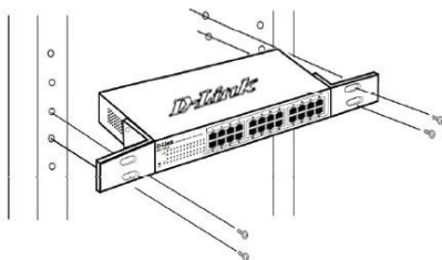
Abbildung 3: Switch im Standardrack installieren
