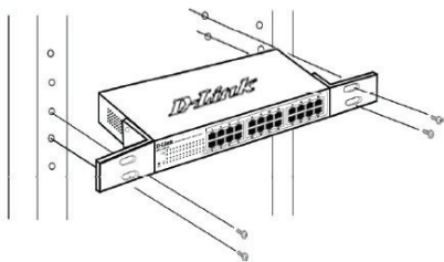
Figure 3. Installation du switch dans une armoire de taille standard
