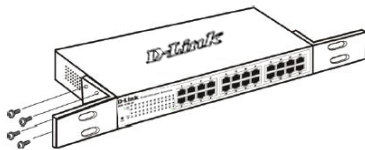
Abbildung 2: Einbauwinkel anbringen
