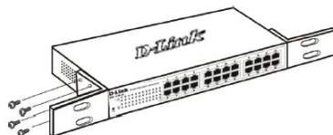
Figura 2. Fixando as braçadeiras de montagem
