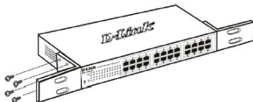
Figura 2. Fijar los ángulos de montaje
