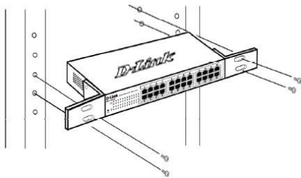
Figura 3. Installazione dello switch all'interno del rack
