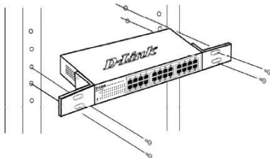
Gambar 3. Memasang switch ke rak dengan ukuran standar
