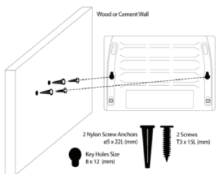
Abbildung 4. Desktop-Switch - Wandmontage
