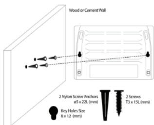
Рисунок 4. Крепление настольного коммутатора к стене
