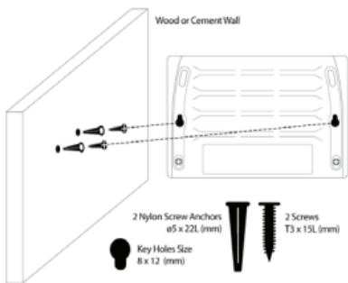
Gambar 4. Memasang switch ke dinding
