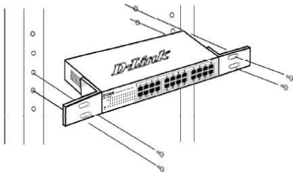
Рисунок 3. Установка коммутатора в стандартную стойку
