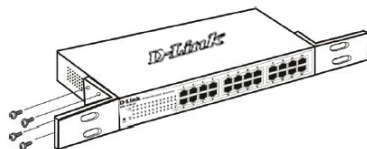
Figure 2. Fixation des supports de montage
