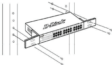
圖 3. 安裝交換器到標準尺寸的機架
