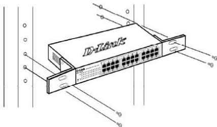
Figura 3. Instalar el switch en un rack estándar
